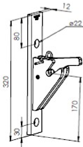
Väggfäste 831300
